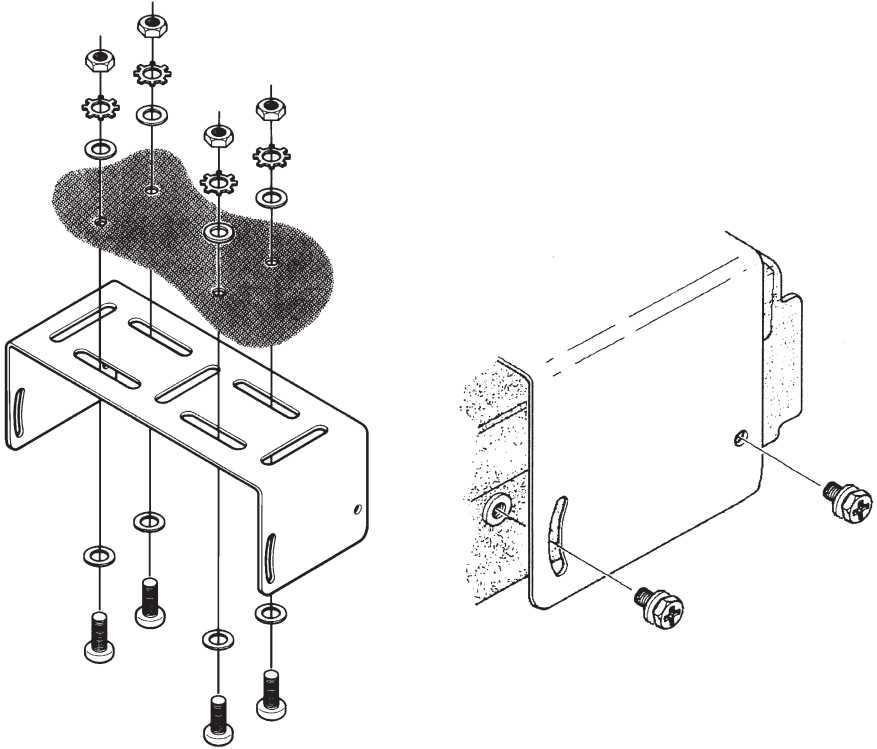
安装 MMB-36
